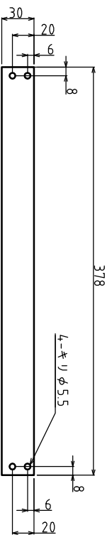
プレートC ステンレス薄板未研磨品 (2B) シヤーリング切断 t=0.8mm
