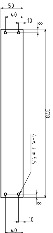
プレートB ステンレス薄板未研磨品 (2B) シヤーリング切断 t=0.8mm
